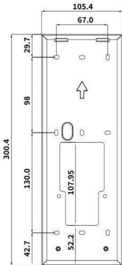
① 正视图 Front view
