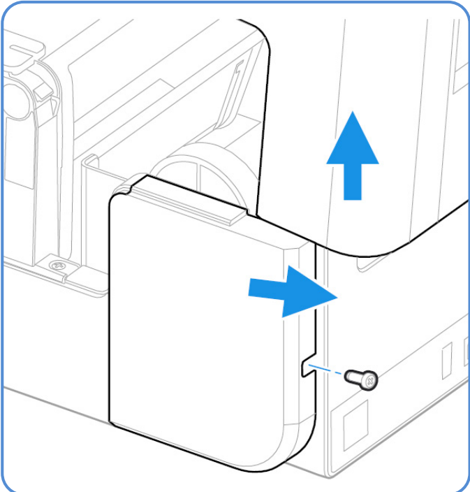
PC42E-T - Wi-Fi/BT Module Door
