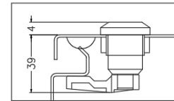
DOOR LOCK DOOR LOCK DIMENSIONS
