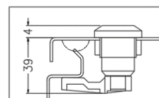
DOOR LOCK
