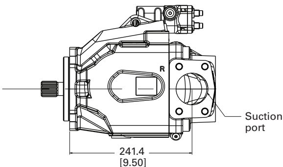
View A-A
